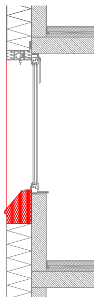
Systemskizze Sohlbankprofil
