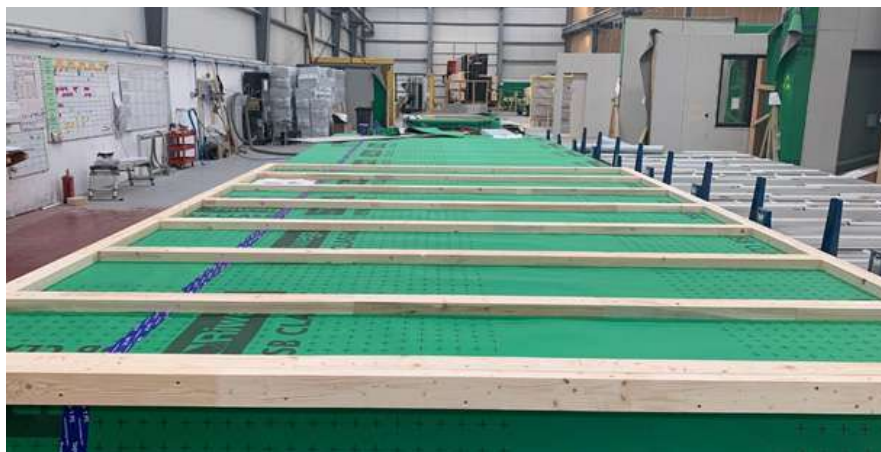
Figura 10. Imagen en taller (Fuente: Medgón PassivHaus)
