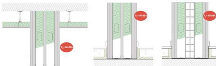
EJEMPLOS DE TIPOLOGÍA DE AISLAMIENTO ACÚSTICO
